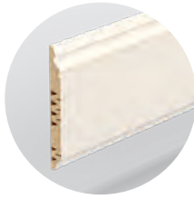
Beschilderbare Ogee-plint QSISKROGEE 2.400 x 16 x 160 mm
